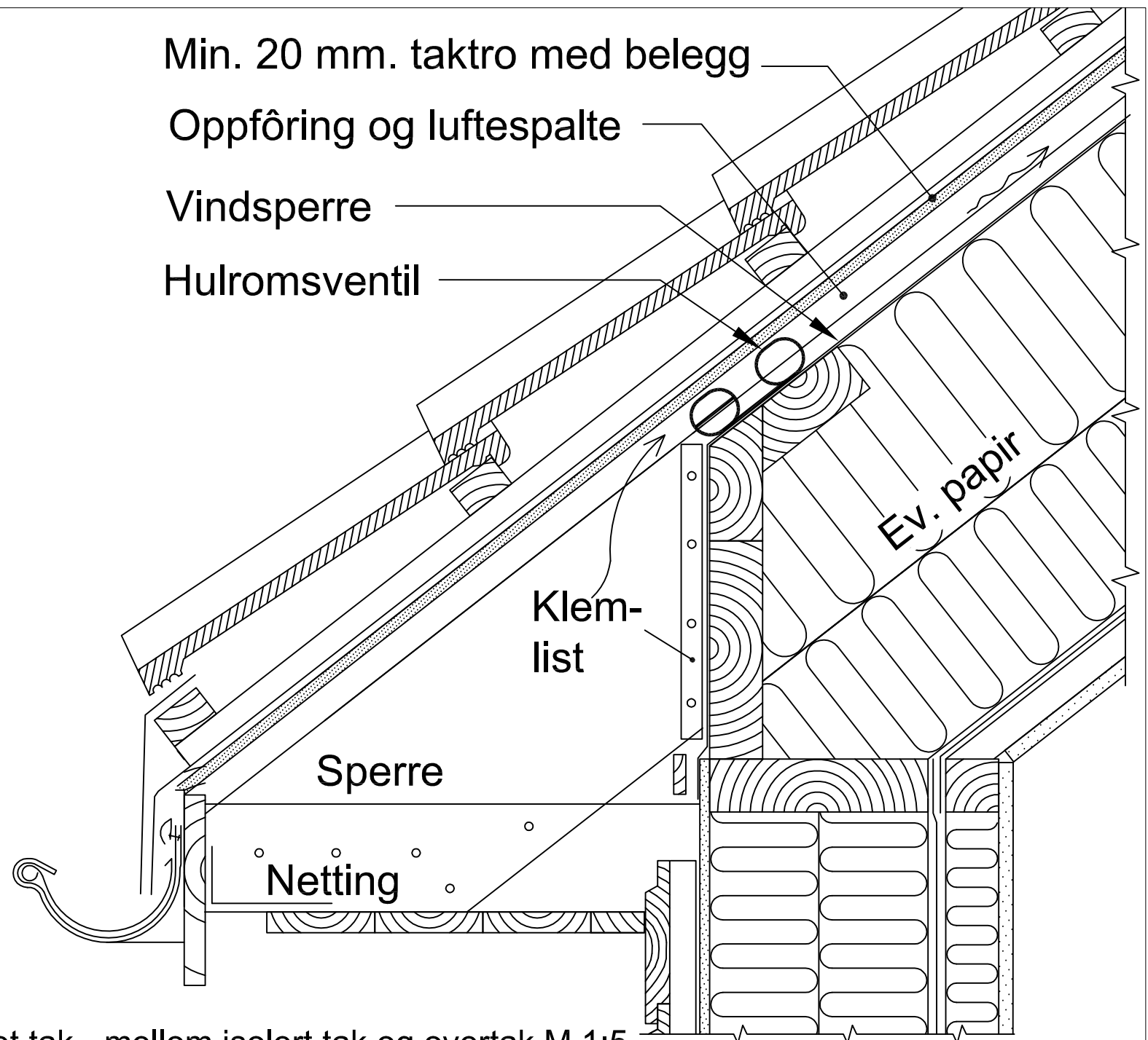
Montering i luftet tak - mellom isolert tak og overtak M 1:5
