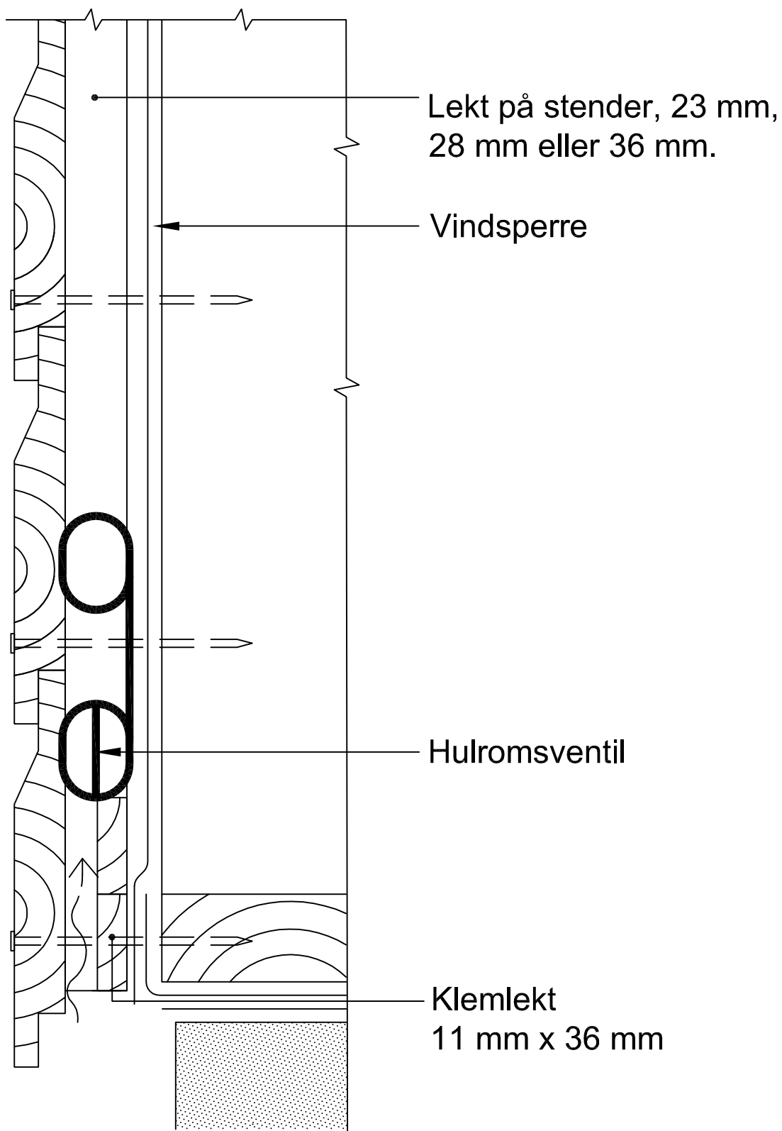
Montering i utlektet horisontal kledning - M 1:2
